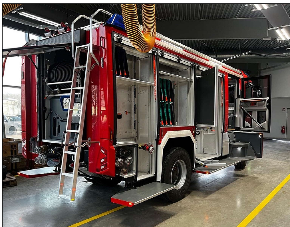
Das neue Einsatzfahrzeug der FF Neidling, HLF3 (Hilfslöschfahrzeug)
